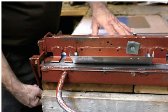
アルミの板を一枚ずつ曲げて、パーツをつくります。 Aluminium plates are individually bent to form each component.
